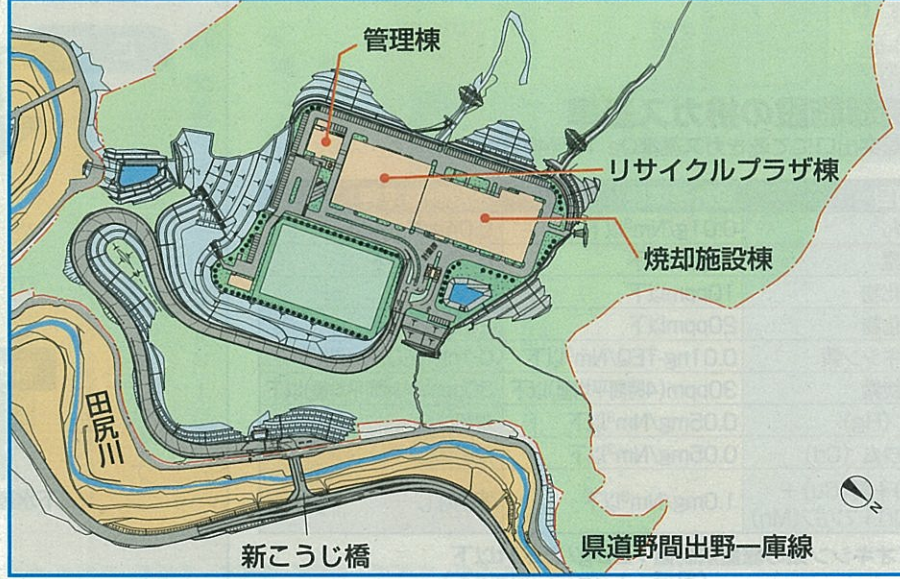
敷地全体配置図
