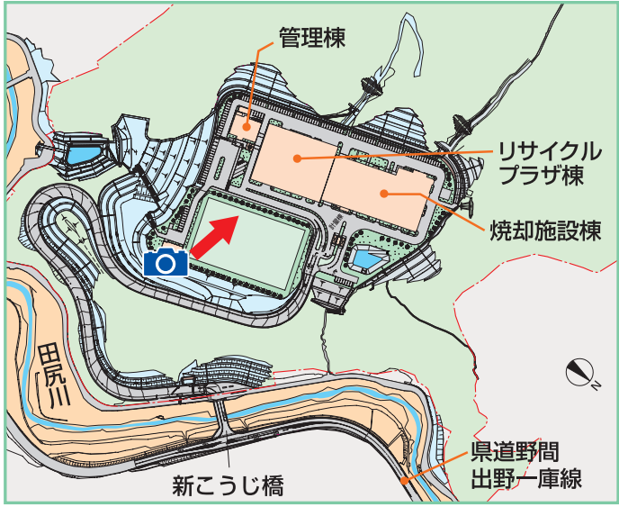
建物配置図
